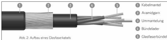
Abb. 2: Aufbau eines Glasfaserkabels
